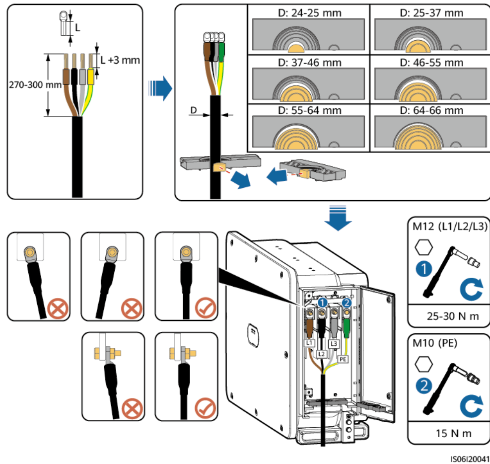
Abbildung 5-12 Kabelanschluss
