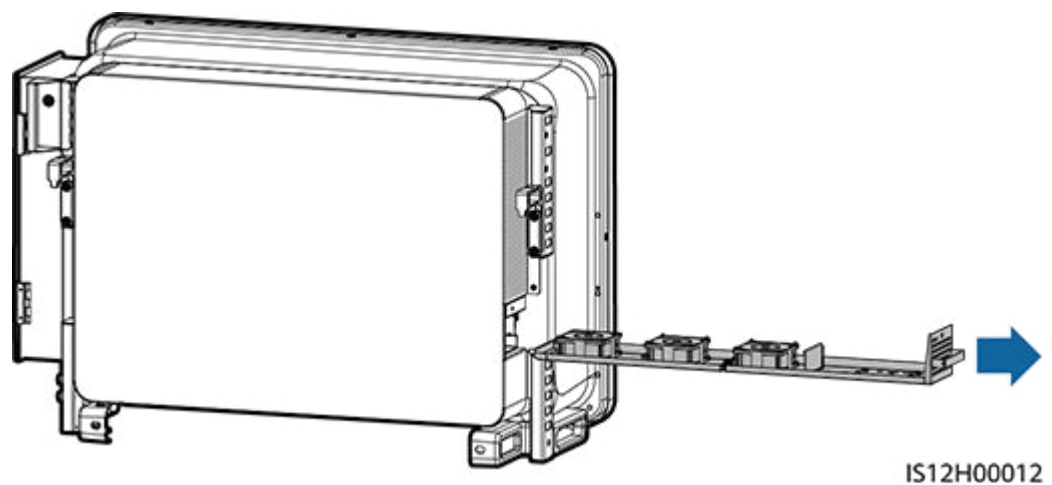
Abbildung 8-5 Herausziehen der Lüfterablage (2)
