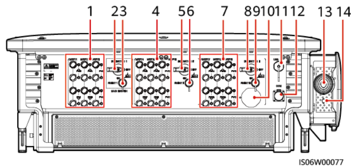
Abbildung 2-5 Abbildung der Anschlüsse (Automatischer DC-Schalter)
