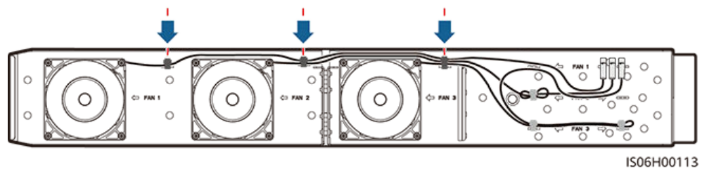
Abbildung 8-11 Zusammenbinden der Kabel für LÜFTER 1
