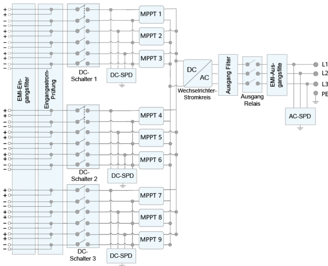
Abbildung 2-7 Konzeptdiagramm des Wechselrichters
