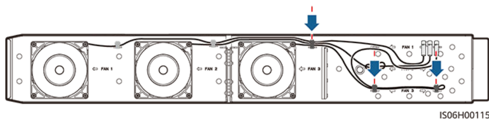
Abbildung 8-13 Zusammenbinden der Kabel für LÜFTER 3
