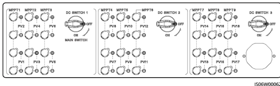
Abbildung 5-15 DC-Klemmen
