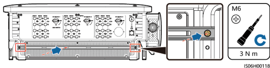
Abbildung A-5 Installieren eines Trägers
