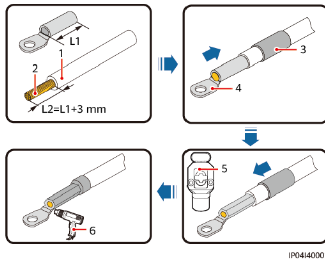
Abbildung 5-4 Crimpen einer DT-Klemme
