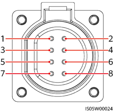
Abbildung 5-20 Kommunikationsanschlüsse
