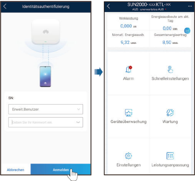
Abbildung 7-6 Anmeldung
