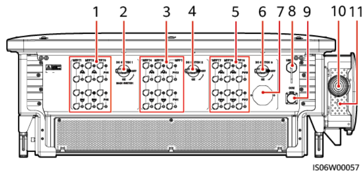
Abbildung 2-4 Abbildung der Anschlüsse (Manueller DC-Schalter)
