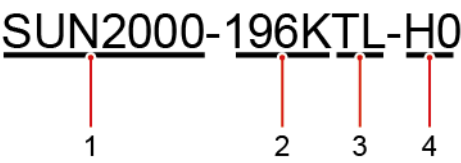
Abbildung 2-1 Modellbeschreibung (SUN2000-196KTL-H0 als Beispiel)
