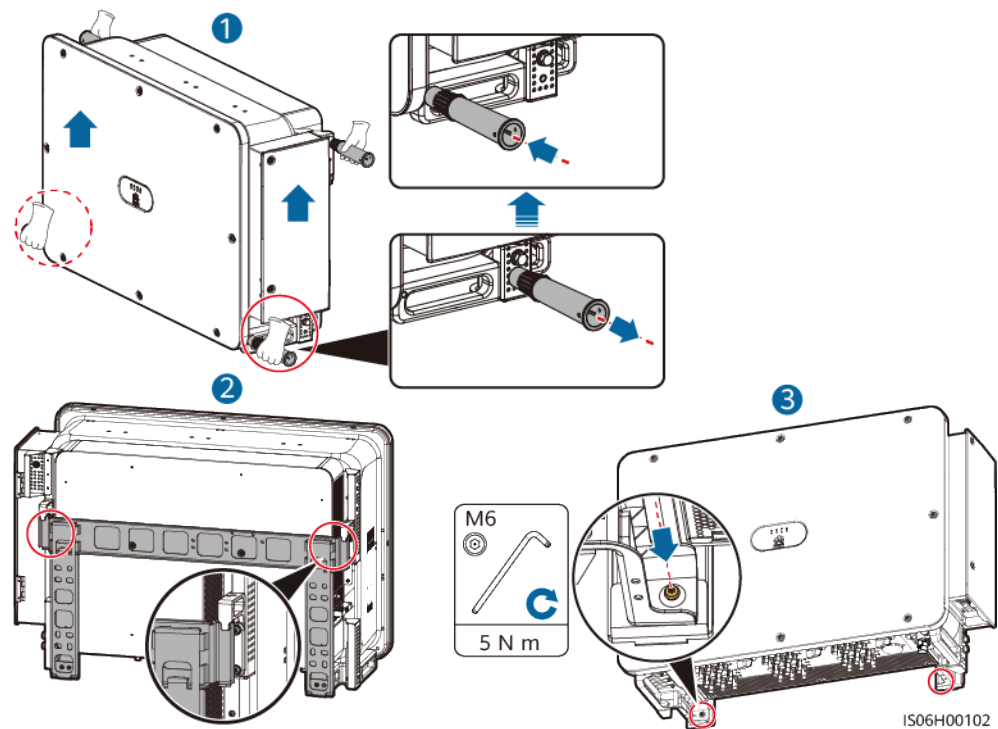
Abbildung 4-13 Montage
