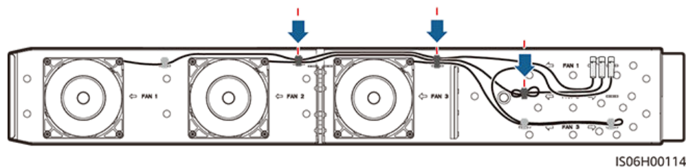
Abbildung 8-12 Zusammenbinden der Kabel für LÜFTER 2
