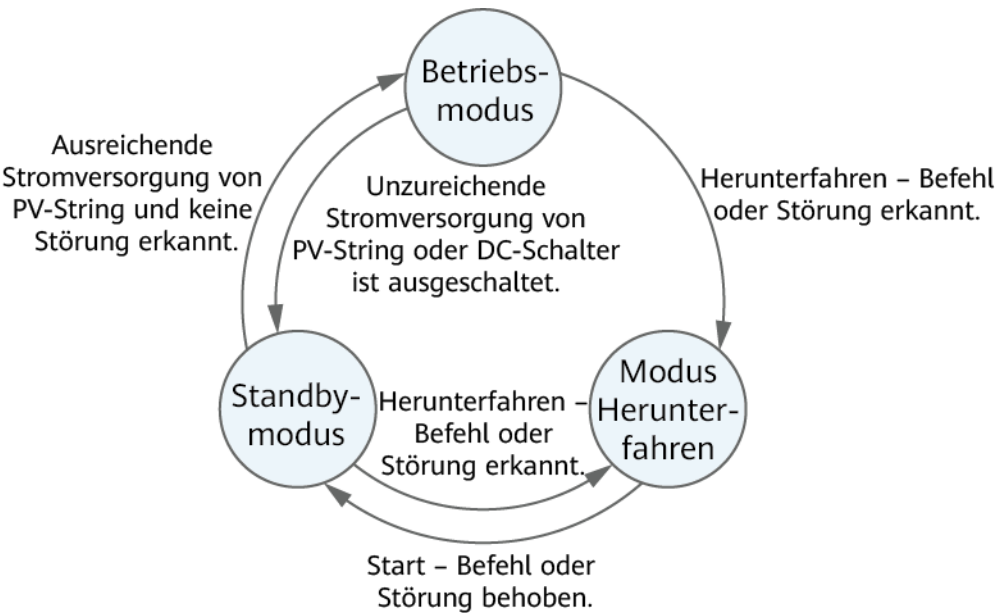
Abbildung 2-8 Arbeitsmodi
