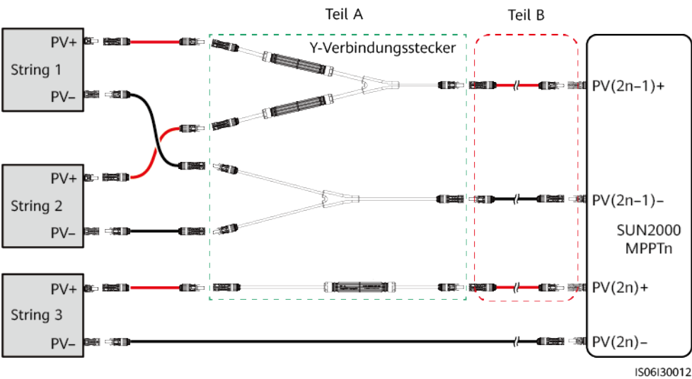
Abbildung 5-16 Verkabelungsbeschreibung von Y-Zweig-Steckern
