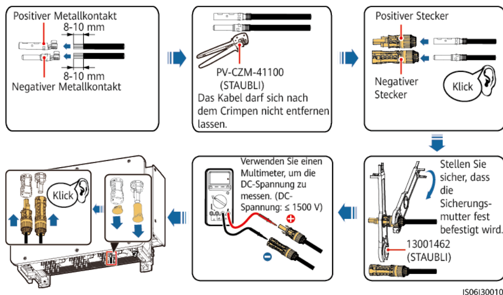
Abbildung 5-17 Kabelanschluss
