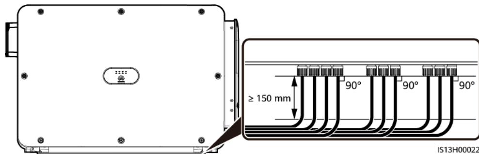
Abbildung 5-19 Anschlussanforderungen für DC-Eingangsstromkabel
