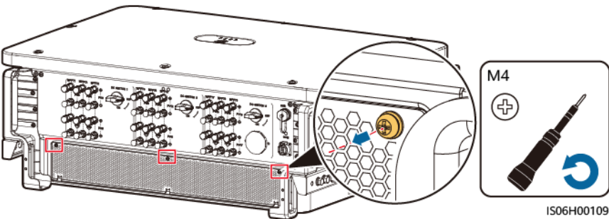
Abbildung 8-2 Entfernen der Trennwand
