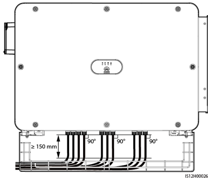
Abbildung A-3 Platzieren der Y-Zweig-Stecker
