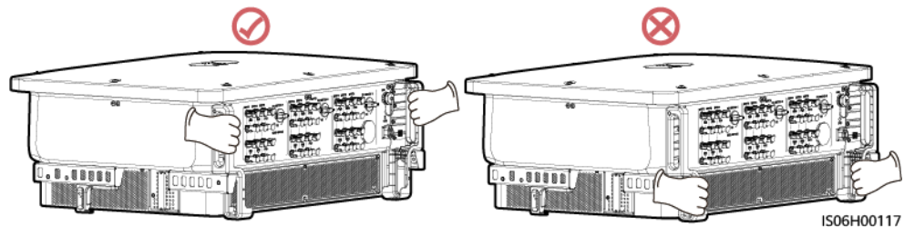
Abbildung 4-12 Hebeposition
