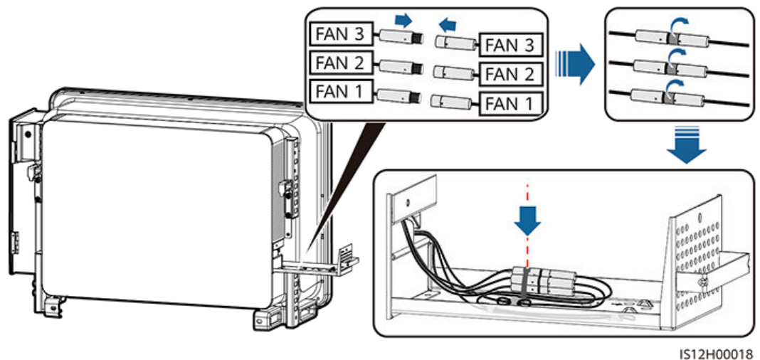
Abbildung 8-15 Neuanschießen und Zusammenbinden der Kabel
