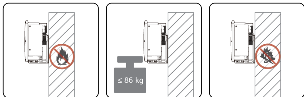
Abbildung 4-1 Montagestruktur
