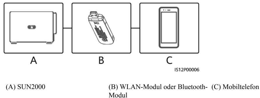
Abbildung 7-1 Verbindung über ein WLAN-Modul oder ein Bluetooth-Modul
