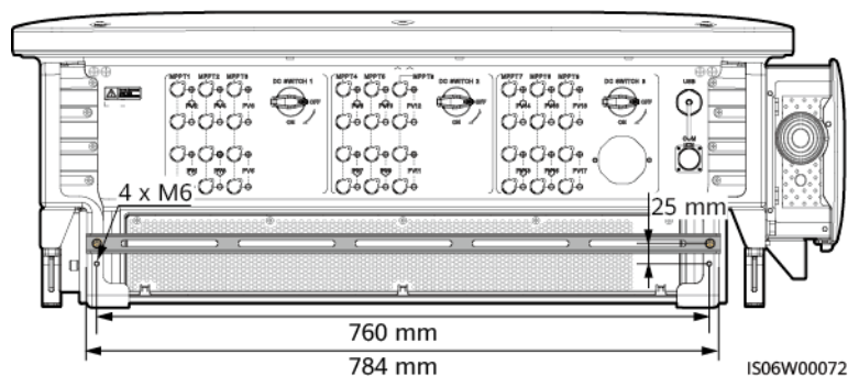
Abbildung A-4 Empfohlene Abmessungen
