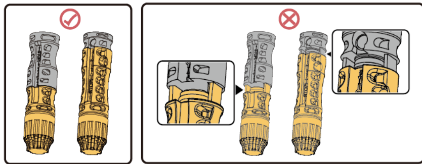
Abbildung 5-18 Anschluss der Steckverbinder
