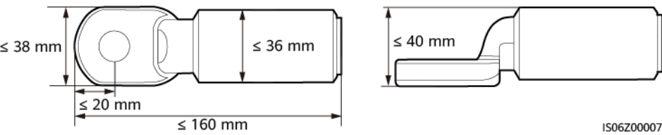
Abbildung 5-9 Spezifikationen der gecrimpten Kabelschuh-/DT-Klemme
