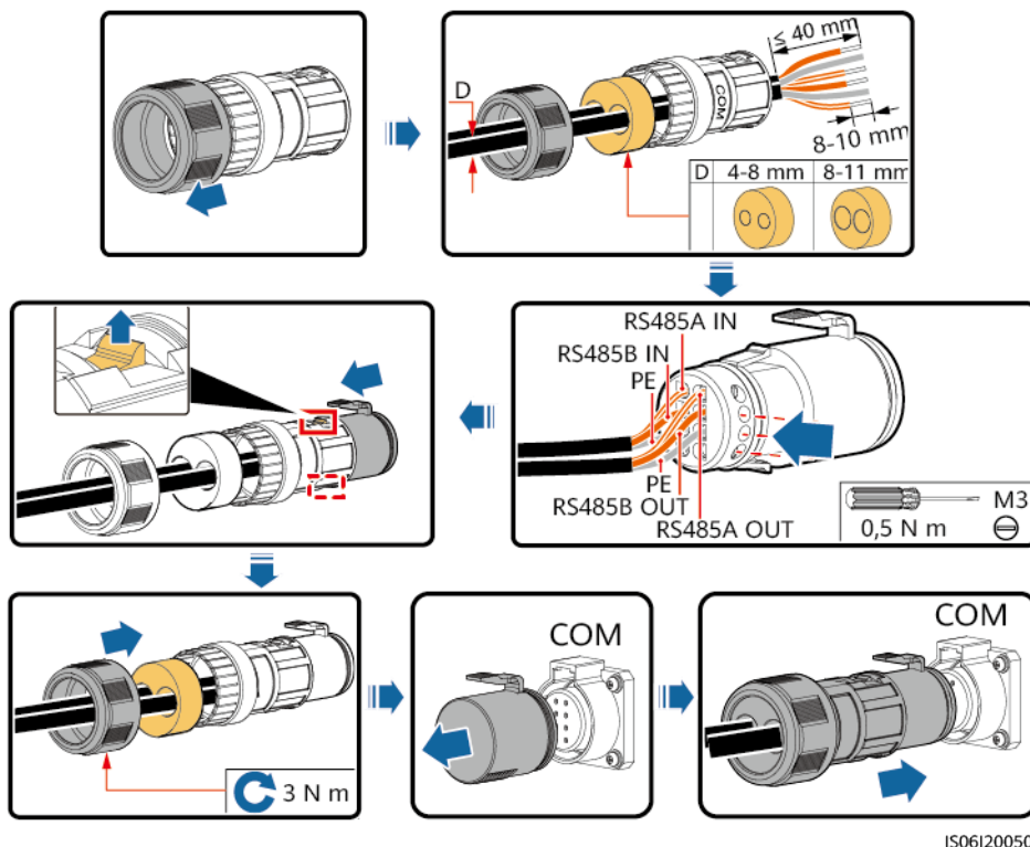
Abbildung 5-22 Kabelverbindung (zweilöchriger Gummistöpsel 4-8 mm)
